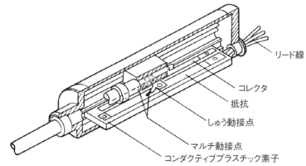
※図-2: 直線形の内部構造例(LP-F シリーズ)
