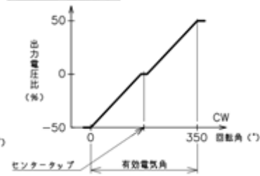
Bタップ出力特性図
