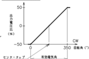
Aタップ出力特性図
