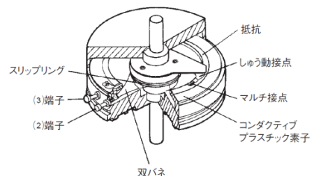
※図-1: 回転形の内部構造例(CPP-45)
